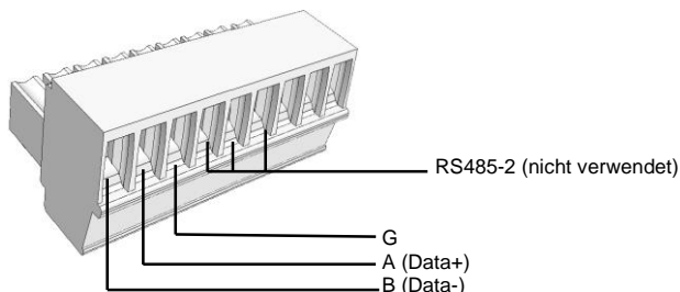
Abbildung 22: RS485 -Klemmleiste
