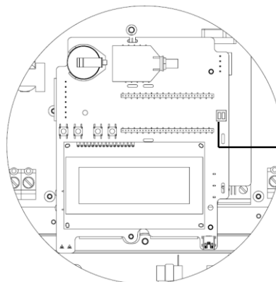
Abbildung 24: RS485 DIP-Schalter
